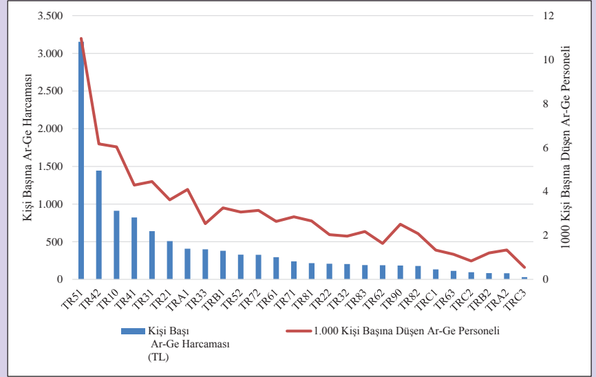
Grafik 1. Düzey 2 Bölgeleri Kişi Başına Düşen Ar-Ge Harcaması ve 1.000 Kişi Başına Düşen Ar-Ge Personeli
