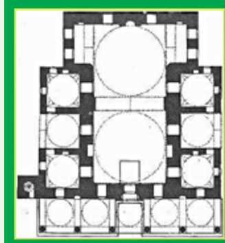
Gedik Ahmet Paşa Camii'nin Planı (M. Baha TANMAN, İslam Ansiklopedisi)
